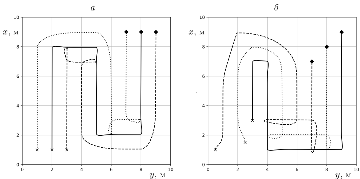
Рис. 6. Траектории роботов при моделировании движения строем: в линию (а) и уступом (б) Fig. 6. Motion trajectory for formation: in a line (a) and a ledge (b)
