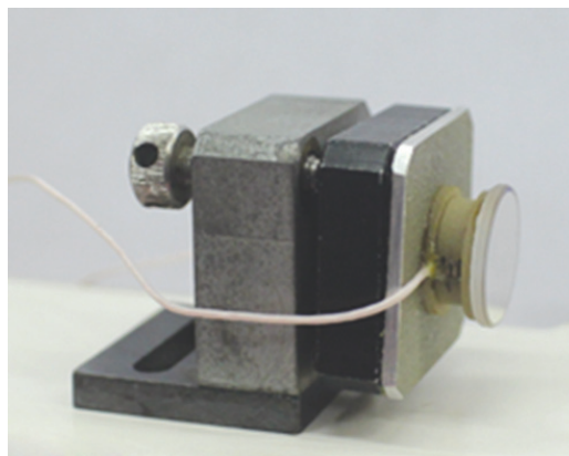
Рис. 3. Опорное зеркало на пьезокерамике
