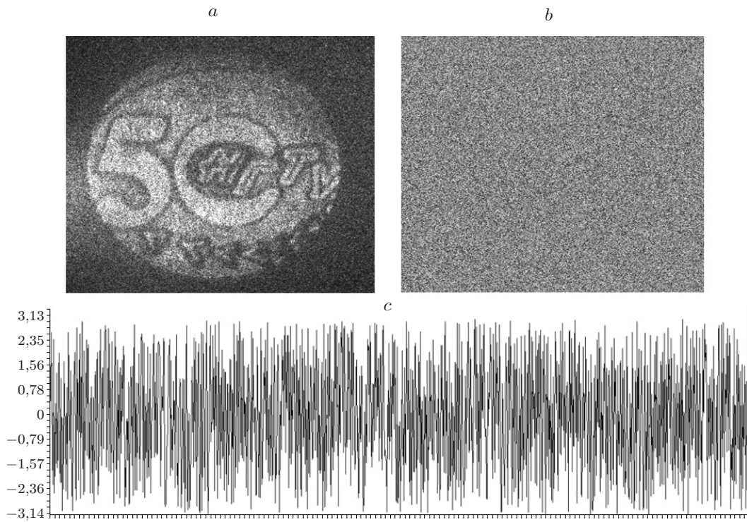
Рис. 2. Восстановленные по цифровой голограмме: амплитуда (а) и фаза (b) объекта; график фазы по центральной строке (с)
