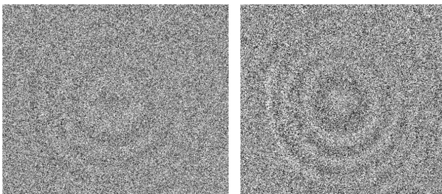
Рис. 7. Цифровые голографические интерференционные картины при различной нагрузке металлической мембраны
