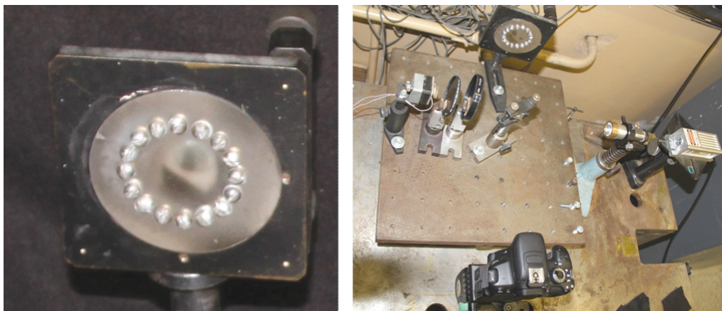
Рис. 6. Фотографии мембраны и оптической установки
