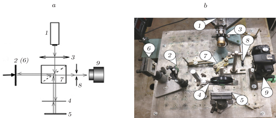
Рис. 1. Схема записи голограммы: схема голографической установки (а); фотография оптической установки (б). Обозначения: 1 — лазер, 2 — объект, 3 — расширитель пучка, 4 — перестраиваемый нейтральный фильтр для изменения уровня интенсивности опорного пучка, 5 — опорное зеркало, 6 — зеркало для юстировки установки, 7 — делитель светового пучка, 8 — диафрагма, 9 — камера
