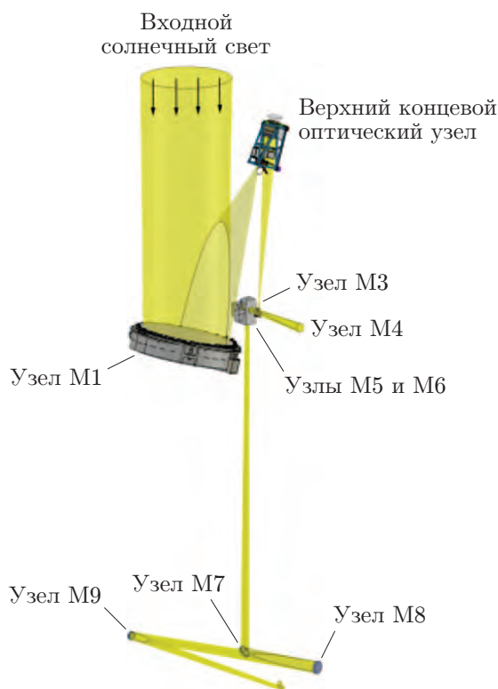
Оптическая схема телескопа DKIST
