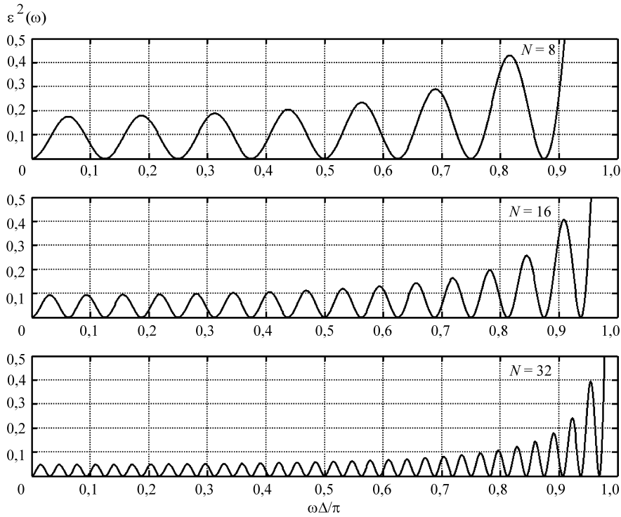
Рис. 3. Дисперсия ошибки реконструкции сигнала формулой (13) при различных значениях числа отсчетов на периоде сигнала
