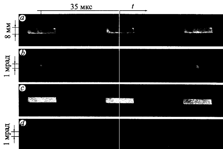
Рис. 6. Покадровые развертки распределения интенсивности излучения SIP-лазера на кристаллах НЛаМ: a , b – в ближней и дальней зонах при 1,4-кратном превышении накачки над пороговой; c , d – в ближней и дальней зонах при 5-кратном превышении порога
