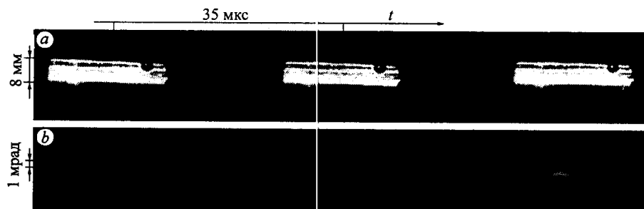
Рис. 5. Покадровые развертки распределения интенсивности излучения SIP-лазера на кристаллах КГВ: a – в ближней зоне (темное пятно – от скола на торце одной из пластин активных элементов); b – в дальней зоне
