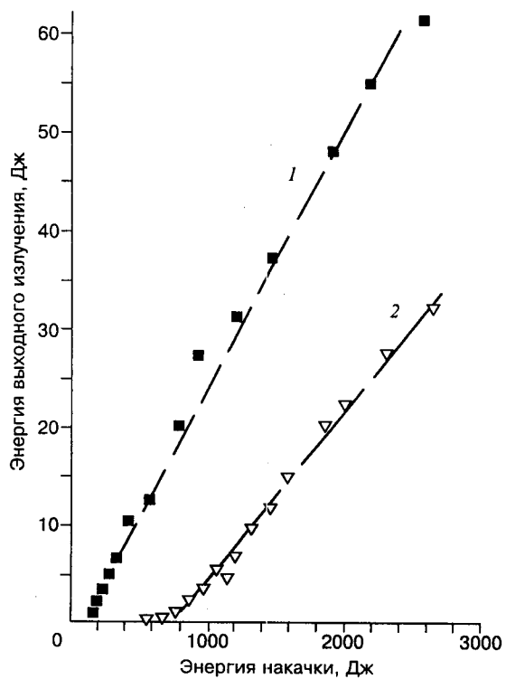
Рис. 3. Зависимость энергии выходного излучения SIP-лазеров от энергии накачки при длительности 1 мс: 1 – КГВ; 2 – НЛЛМ
