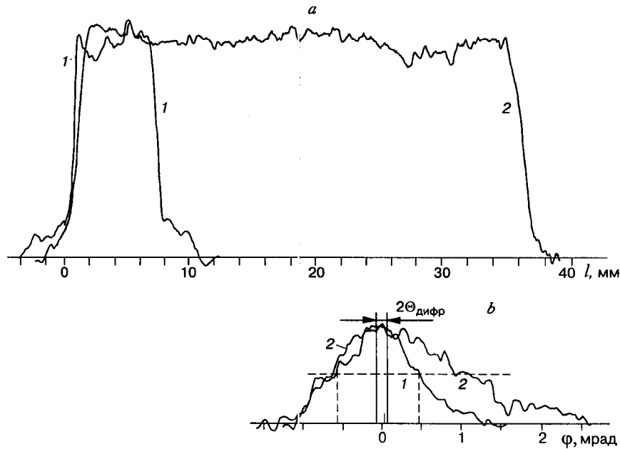
Рис. 7. Денситограммы распределений излучения SIP-лазера на кристаллах НЛaМ: a – на торце пластины активного элемента (1 – поперек и 2 – вдоль ширины пластины); b – по углам (1 – поперек и 2 – вдоль ширины пластины, 2\Theta_{\text{дифр}} указано для толщины пластины 0,8 см)
