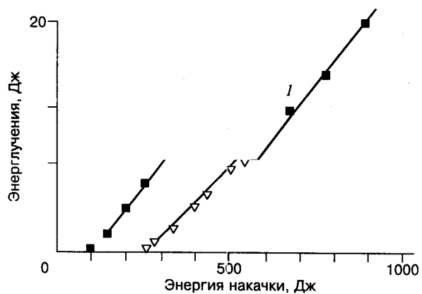
Рис. 2. Зависимость энергии выходного излучения SIP-лазеров от энергии накачки при длительности 180 мкс: 1 – КГВ; 2 – НЛЛМ
