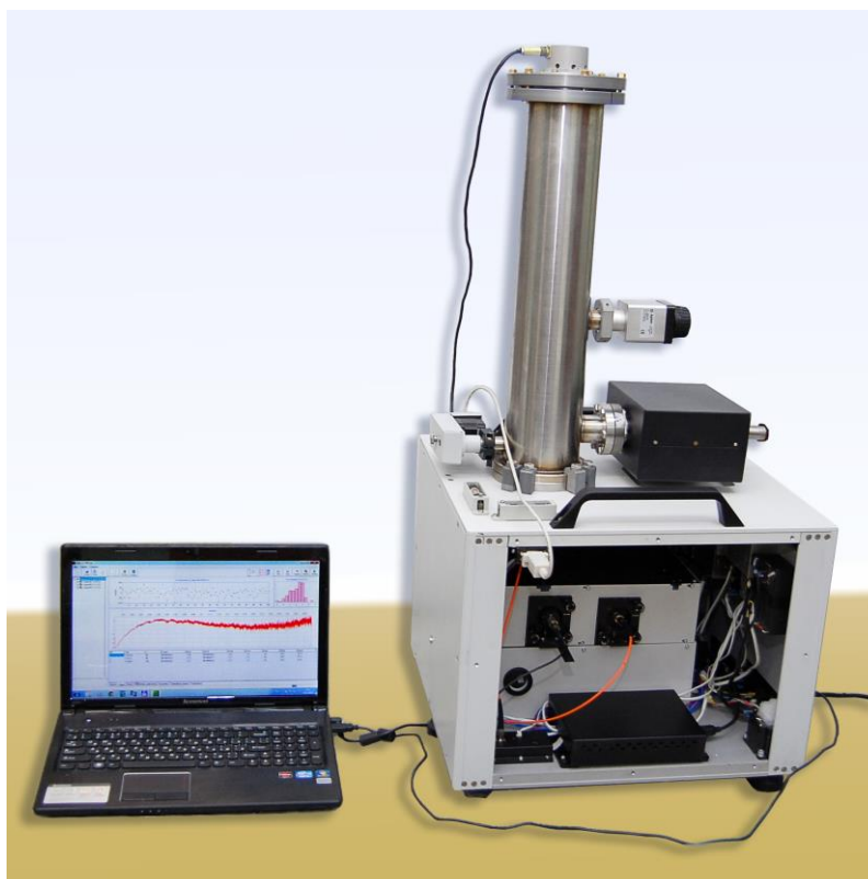
Гравиметр «ГАБЛ-ПМ»
