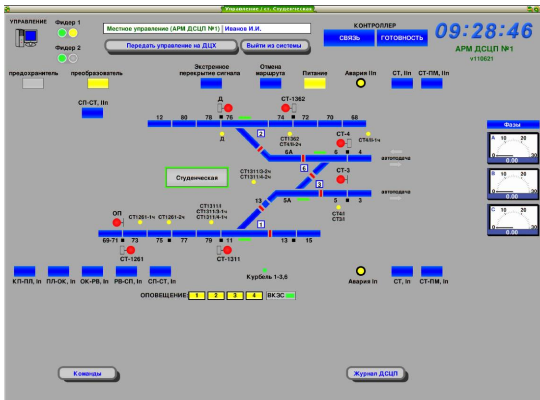
Видеокадр пользовательского интерфейса АСДУ (рабочее место дежурного по станции «Студенческая» Новосибирского метрополитена)
